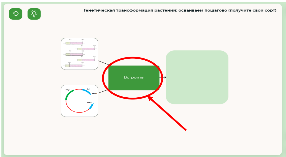
Рис. 5. Встраивание гена
